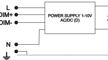
2. Module LED -dimmable power supply (D)
