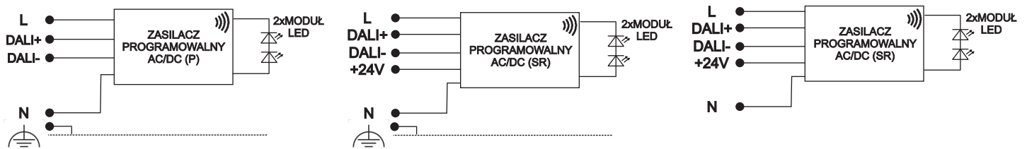
1. Źródło światła LED (I Klasa ochronności) (wersja podstawowa - zasilacz programowalny)
